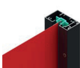
ZIP-Seitenführung Direktmontage
